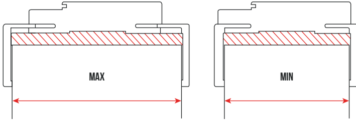
Pervaz Çalışma Payları/Frame Working Margins (0-60 mm)
