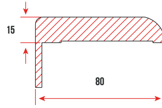
Örnek Pervaz Modeli/Frame Model
